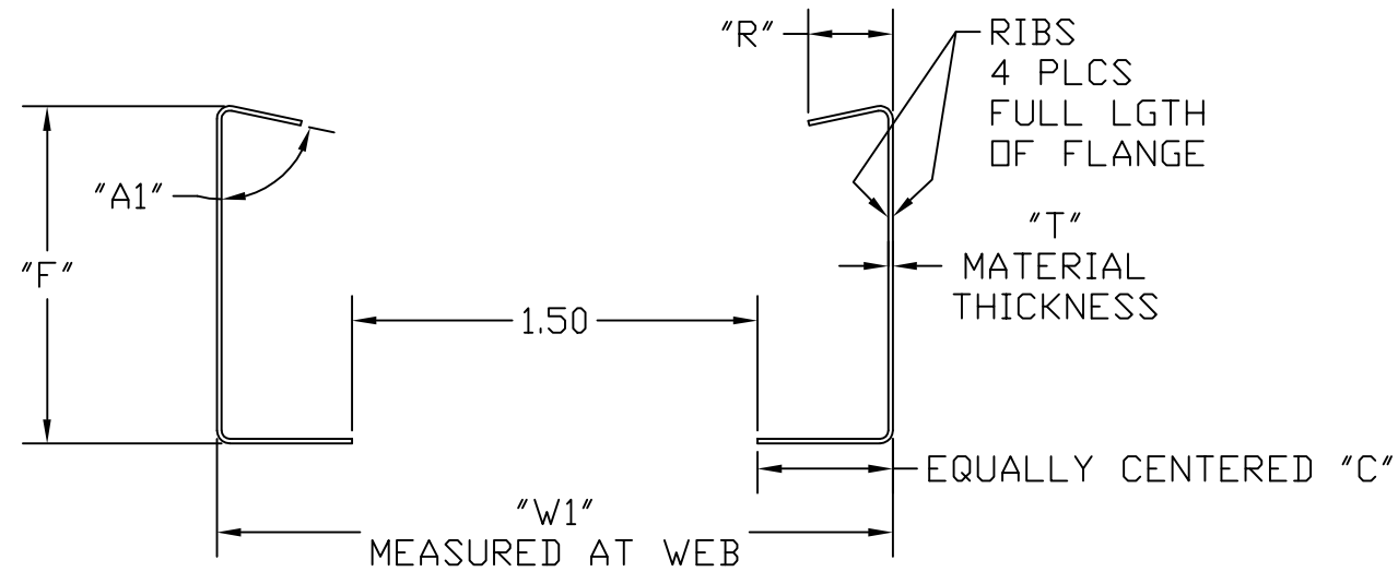
SECT A-A
