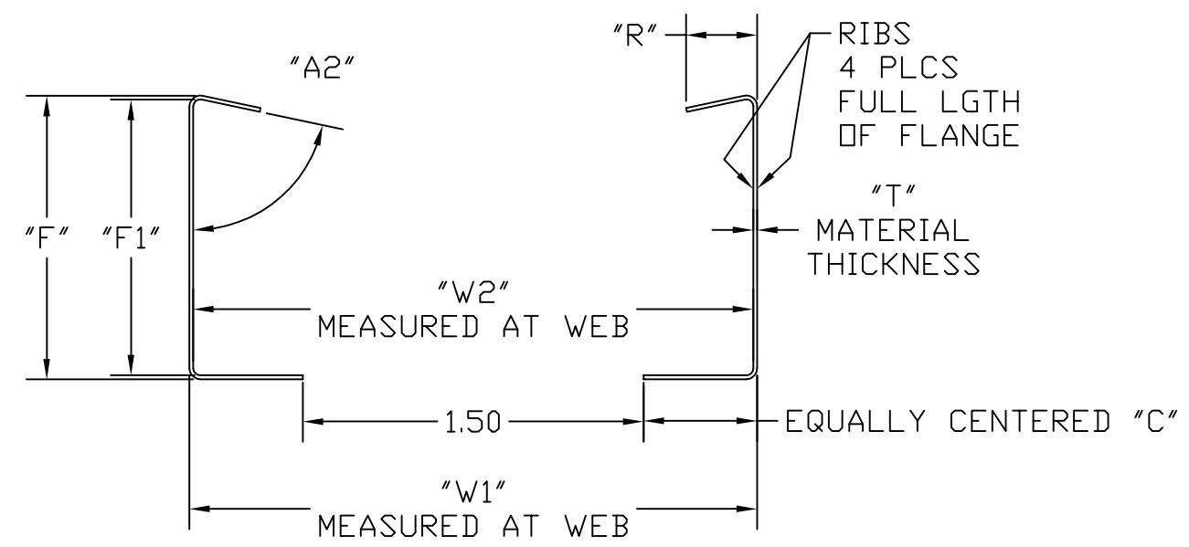
SECT A-A
